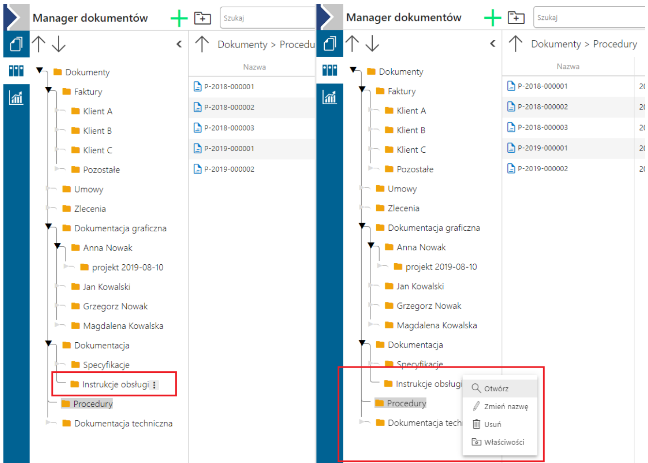
Menu poleceń możliwych do zastosowania na katalogach
