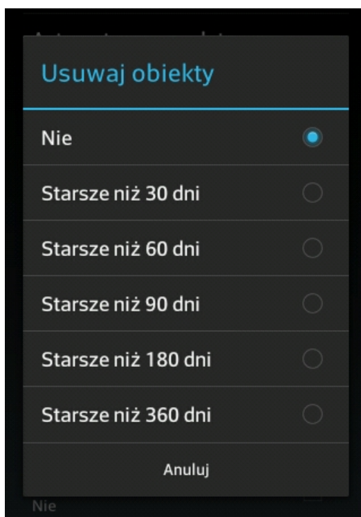
Konfiguracja aplikacji
